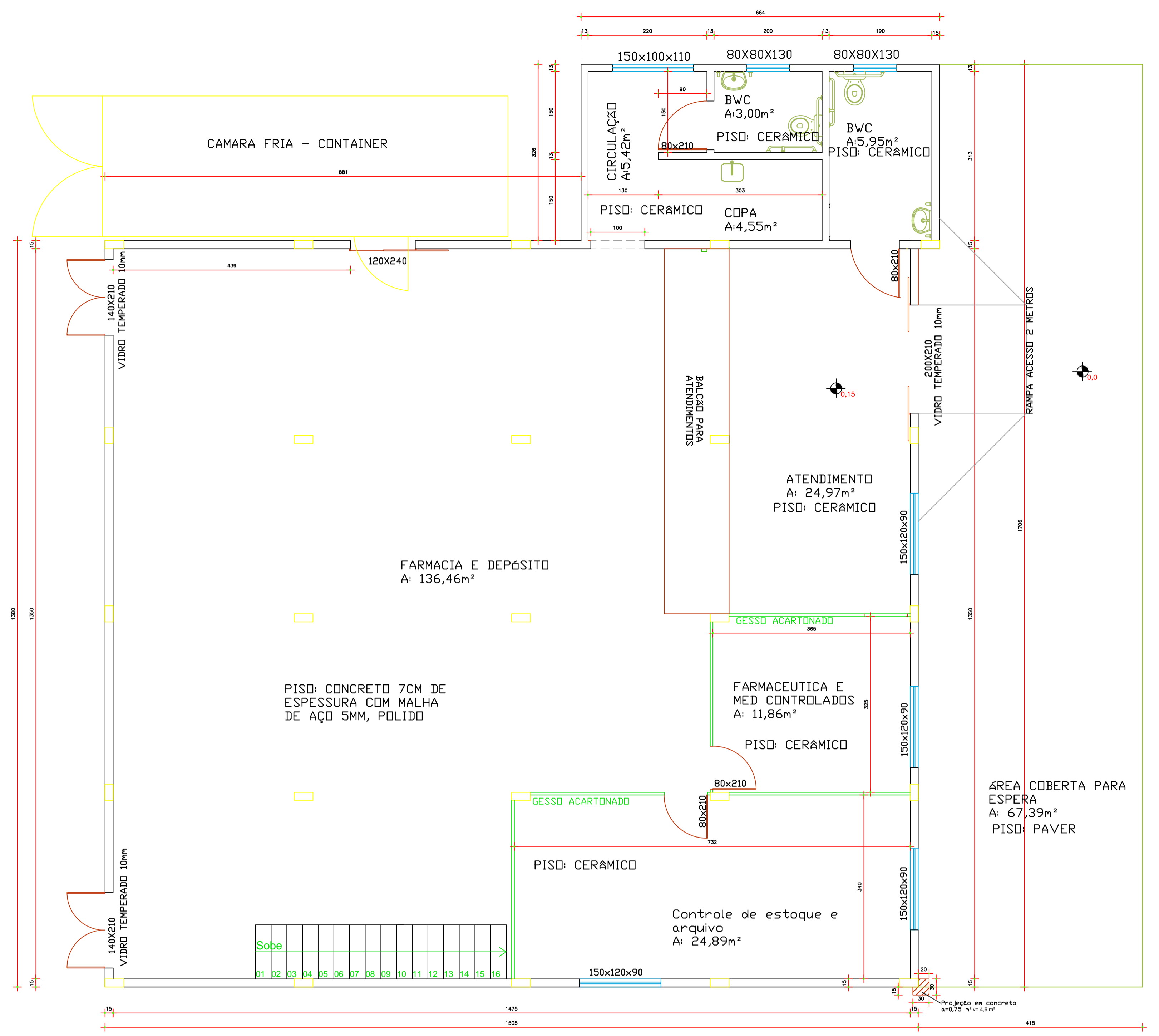
PROJETO ARQUITETONICO TERREO 228 m² ESC. 1 / 50
