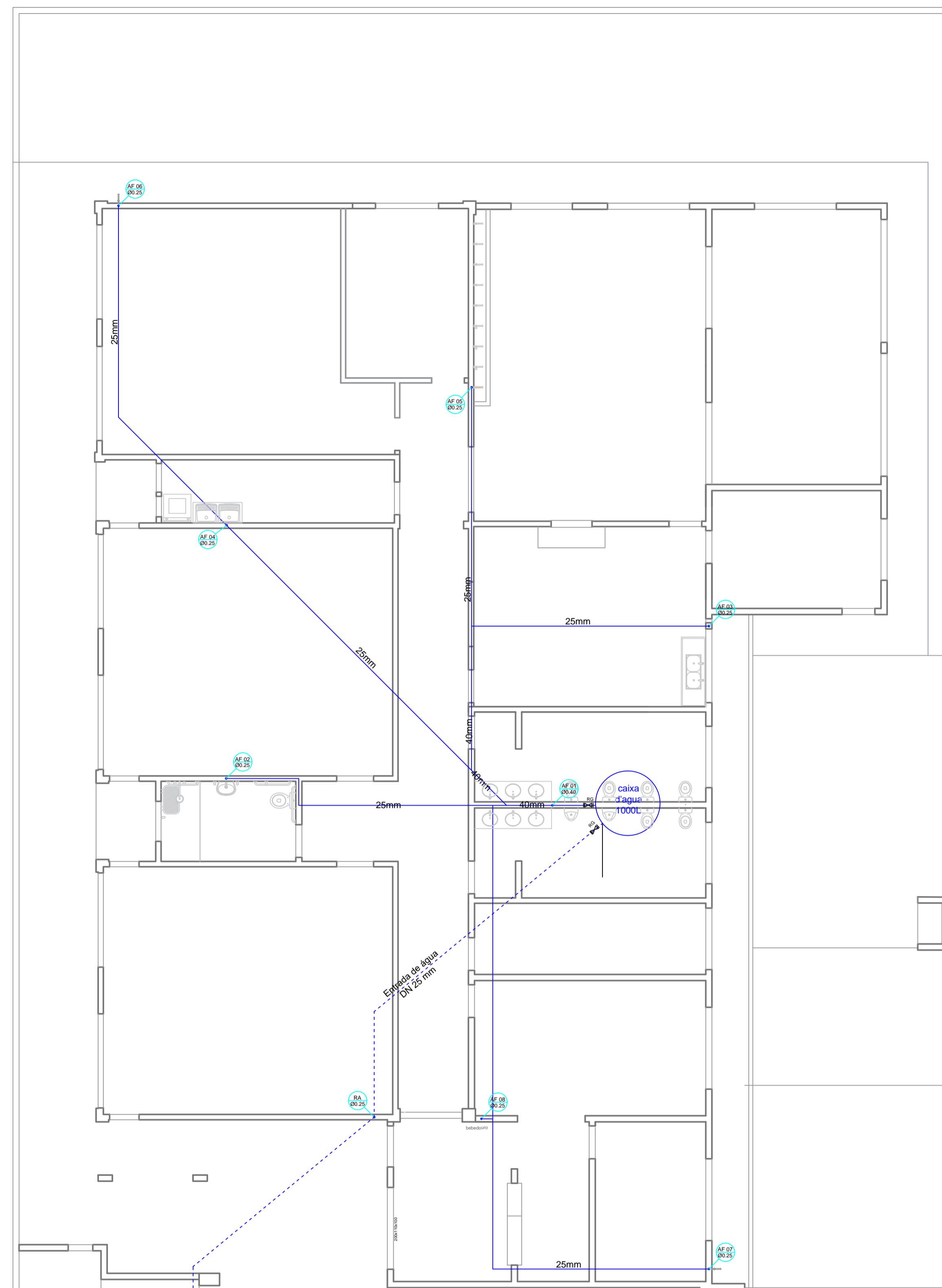
ÁGUA COBERTURA ESCALA 1:50
